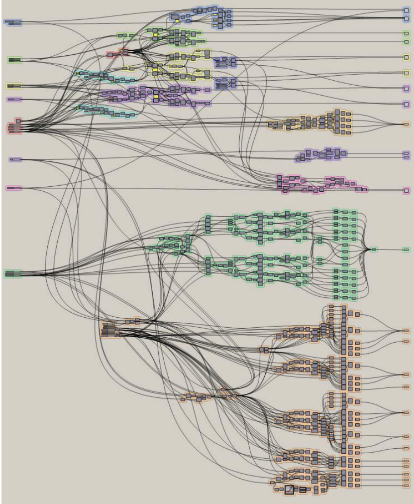
Conception paramétrique, définition Grasshopper
